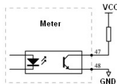
Рисунок 5-3 Импульсный выход
